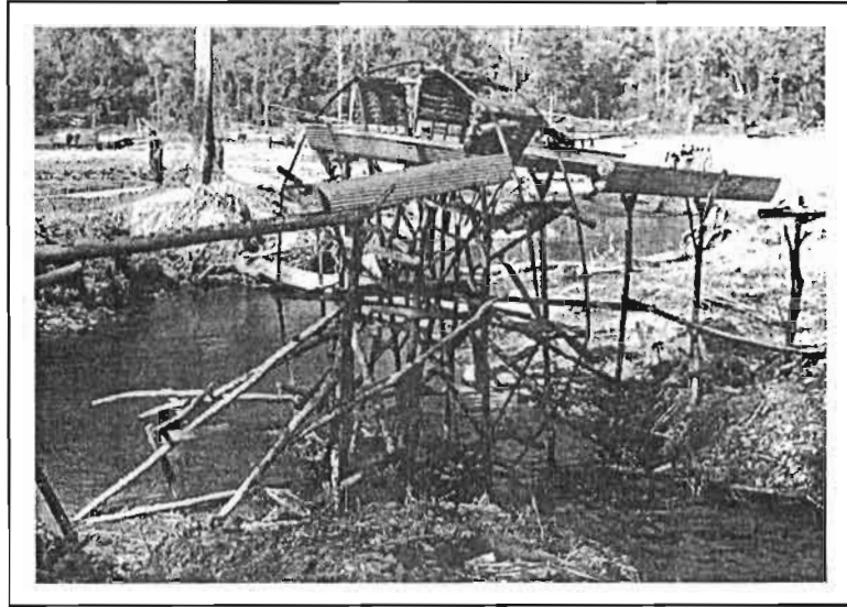
21 กุมภาพันธ์ 2524 วงล้อโพงน้ำตามแบบชนบทอีกแบบหนึ่ง ตามโครงการพระราชดำริ ปางมะผา จังหวัดแม่ฮ่องสอน
