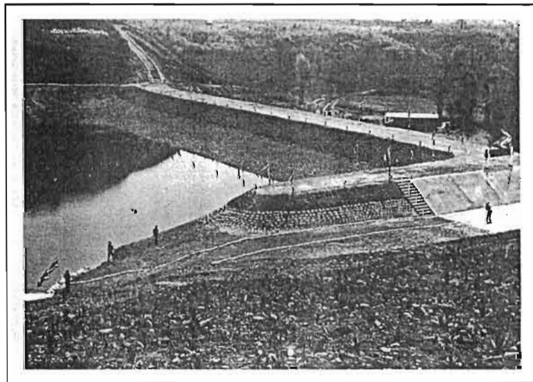
14 กุมภาพันธ์ 2523 โครงการชลประทานในเขตพื้นที่อำเภอทุ่งช้าง จังหวัดน่าน
